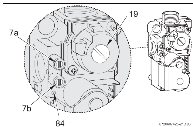
Рис 5 Газовая арматура
