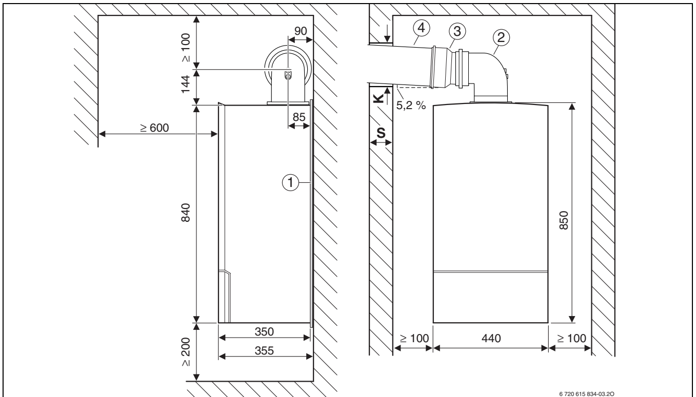
Рис 6 Отвод дымовых газов Ø 100/150 mm
