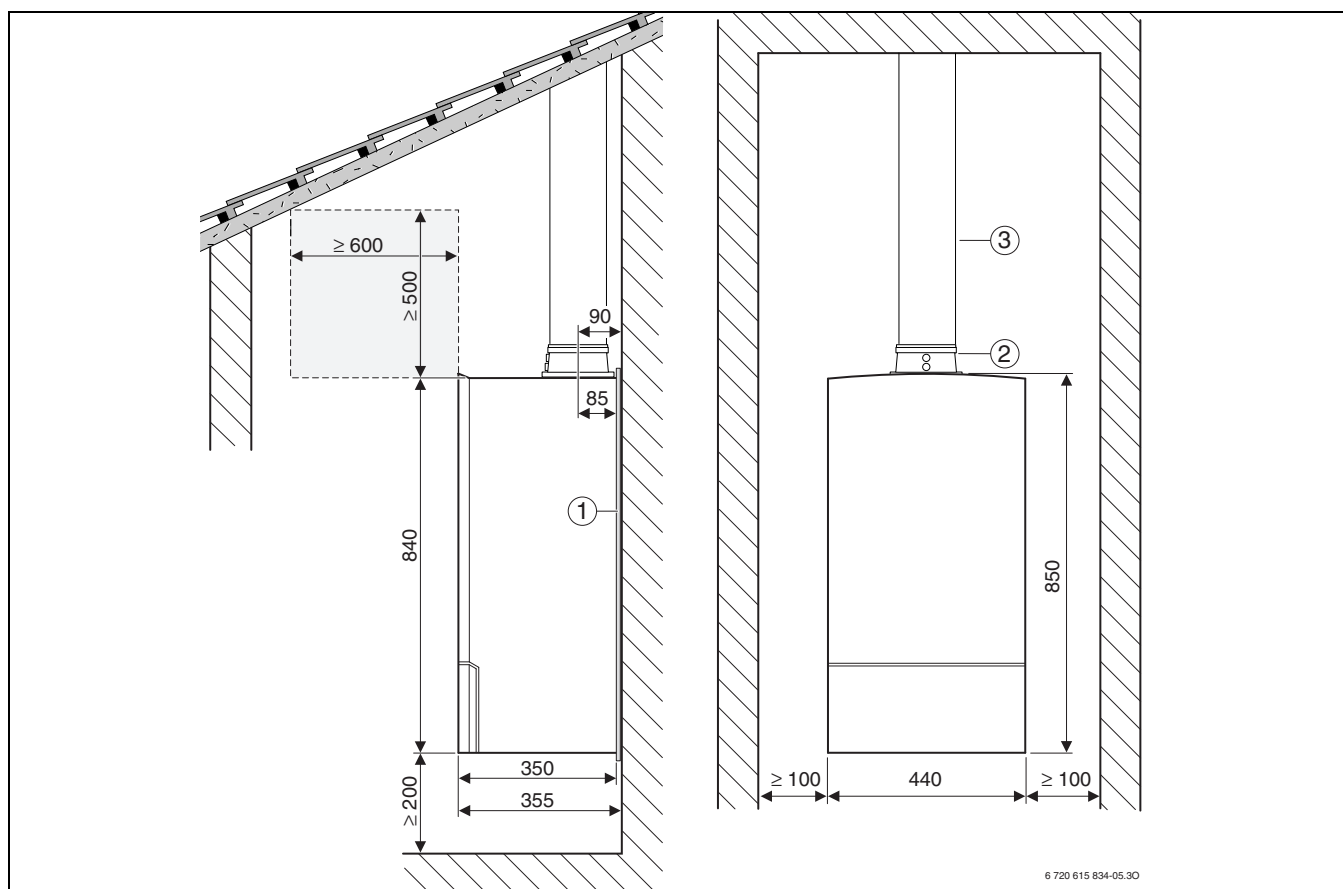
Рис 8 Ø 80/125 мм, наклонная крыша
