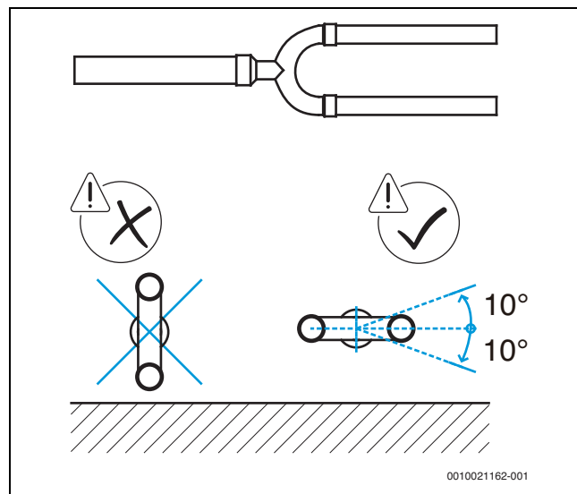
Рис. 15 Расположение U-образного тройникового соединения
