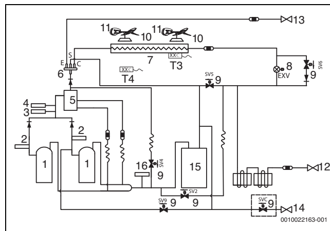
Рис. 54 Схема циркуляции холодильного агента
