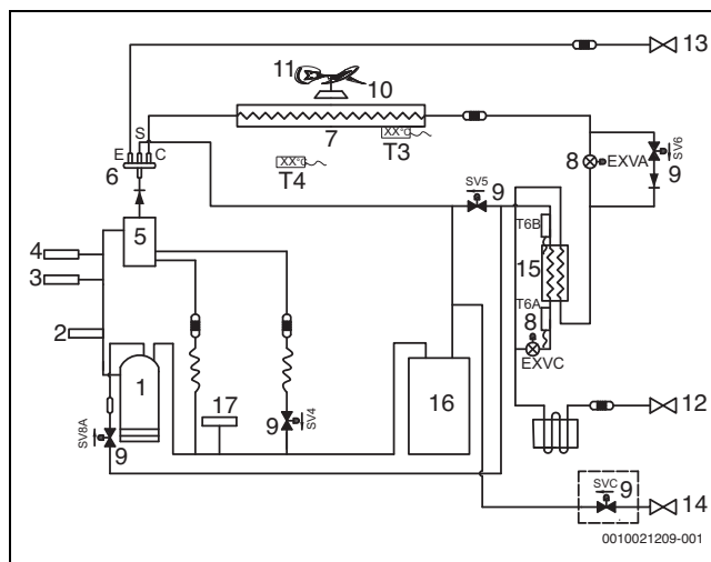
Рис. 50 Схема циркуляции холодильного агента
