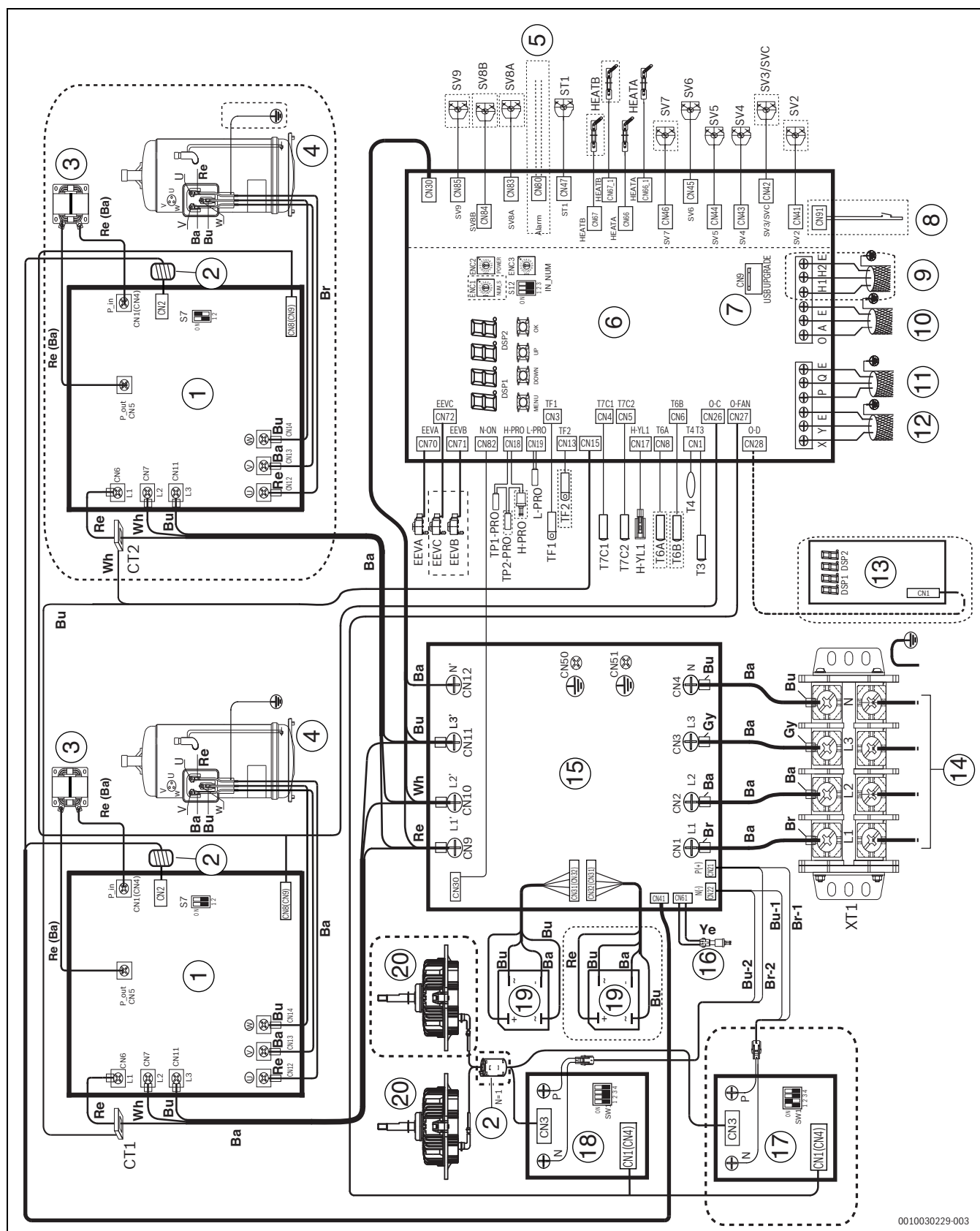
Рис. 73 Электропроводка, модели 8–22 НР
