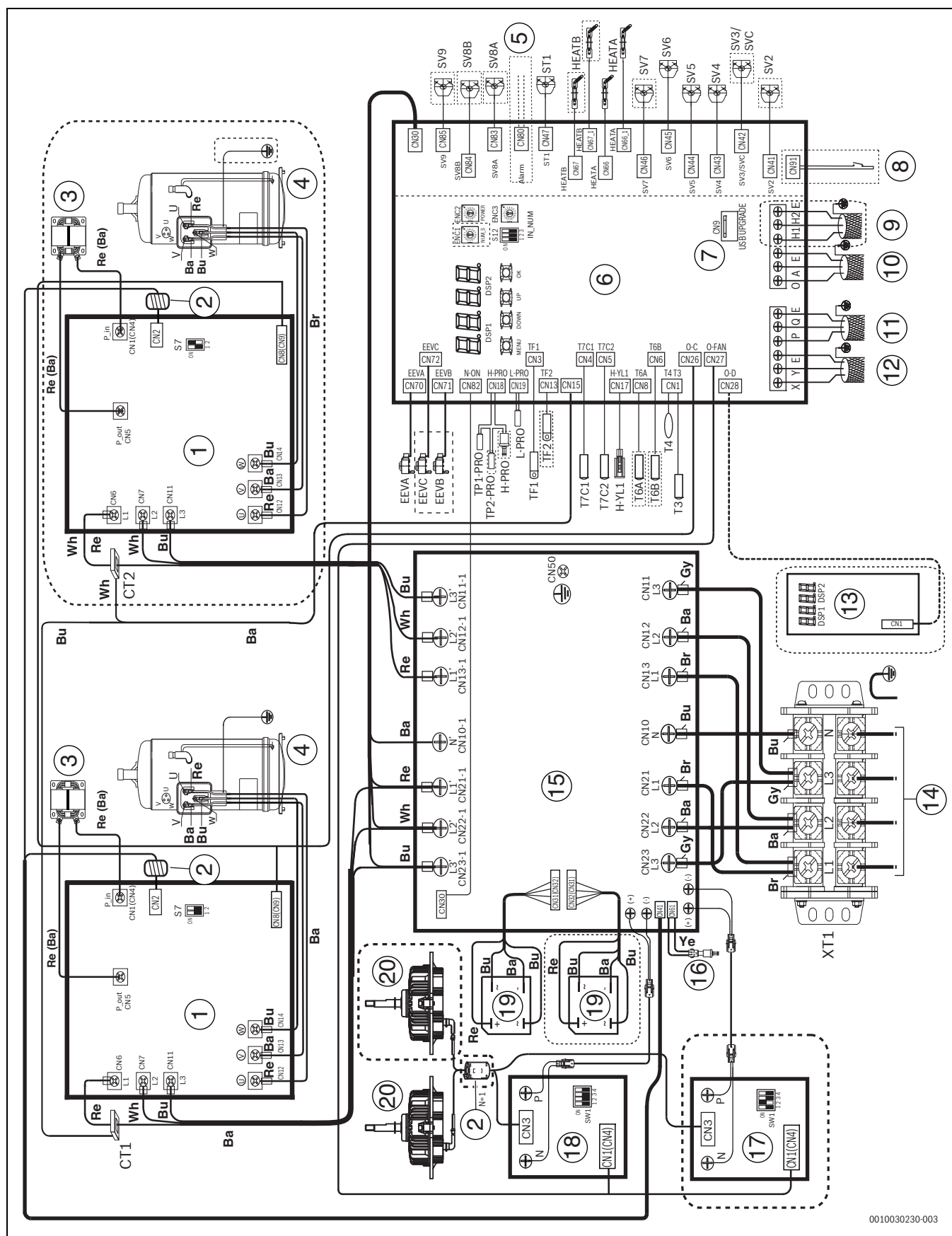
Рис. 75 Электропроводка, модели 24–28 HP
