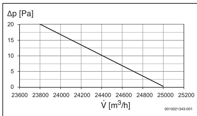
Рис. 64 Производительность вентилятора 2428 НРблоков
