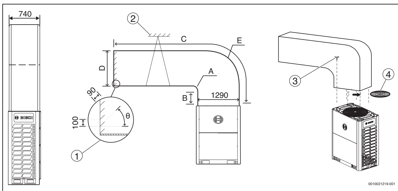
Рис. 69 Опция В: Продольный воздуховод (ед. мм)
