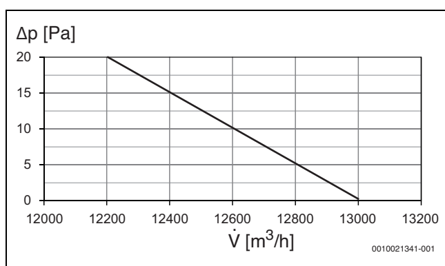
Рис. 62 Производительность вентилятора 1418 НРблоков
