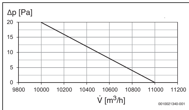
Рис. 61 Производительность вентилятора 812 НРблоков
