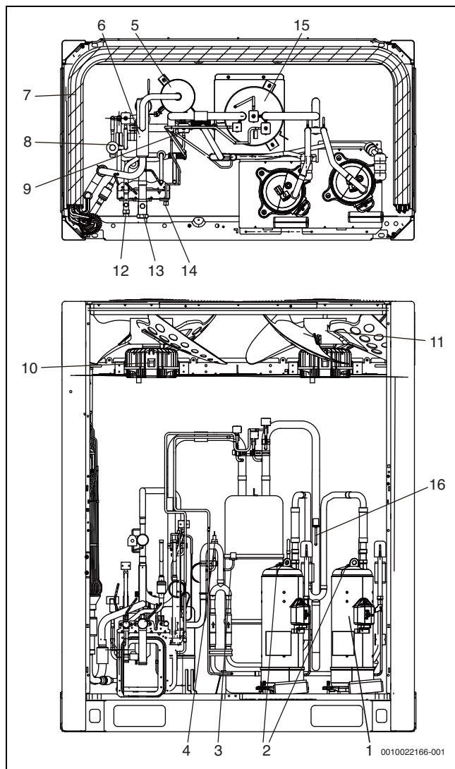
Рис. 53 Расположение компонентов
