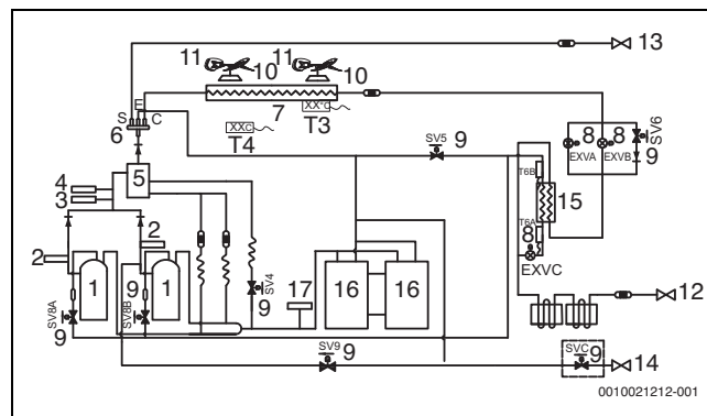
Рис. 58 Схема циркуляции холодильного агента
