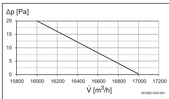
Рис. 63 Производительность вентилятора 2022 НРблоков
