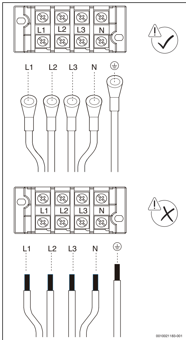
Рис. 34 Электропитание
