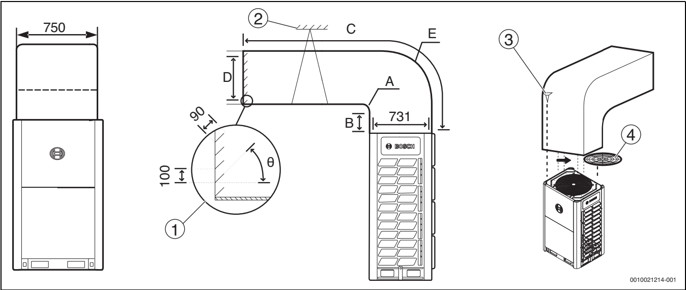
Рис. 66 Опция А: Поперечный воздуховод (ед. мм)
