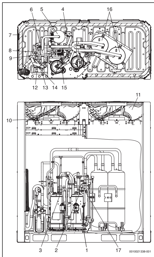
Рис. 59 Расположение компонентов
