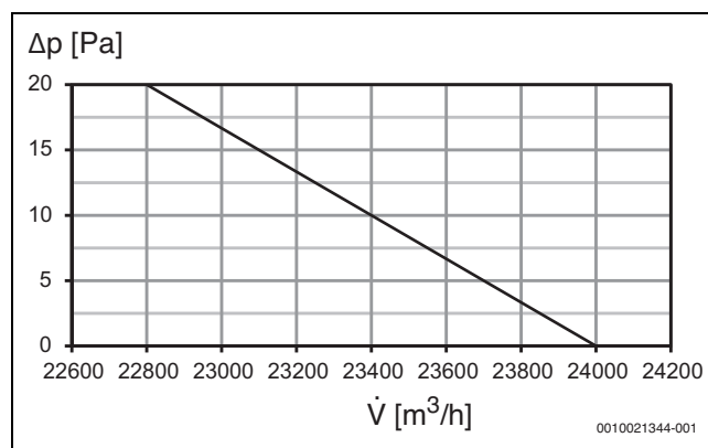
Рис. 65 Производительность вентилятора 3032 НРблоков
