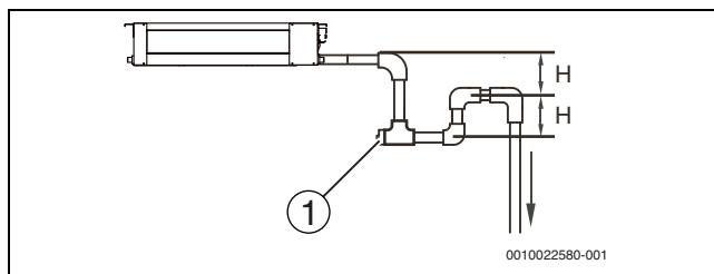
Рис. 19 Схема коленчатого патрубка для сбора воды
