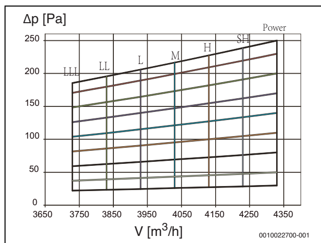
Рис. 30 AF-DH 280-1
