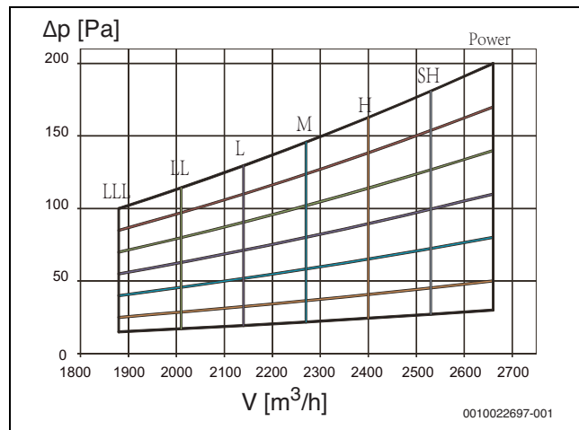
Рис. 27 AF-DH 160-1
