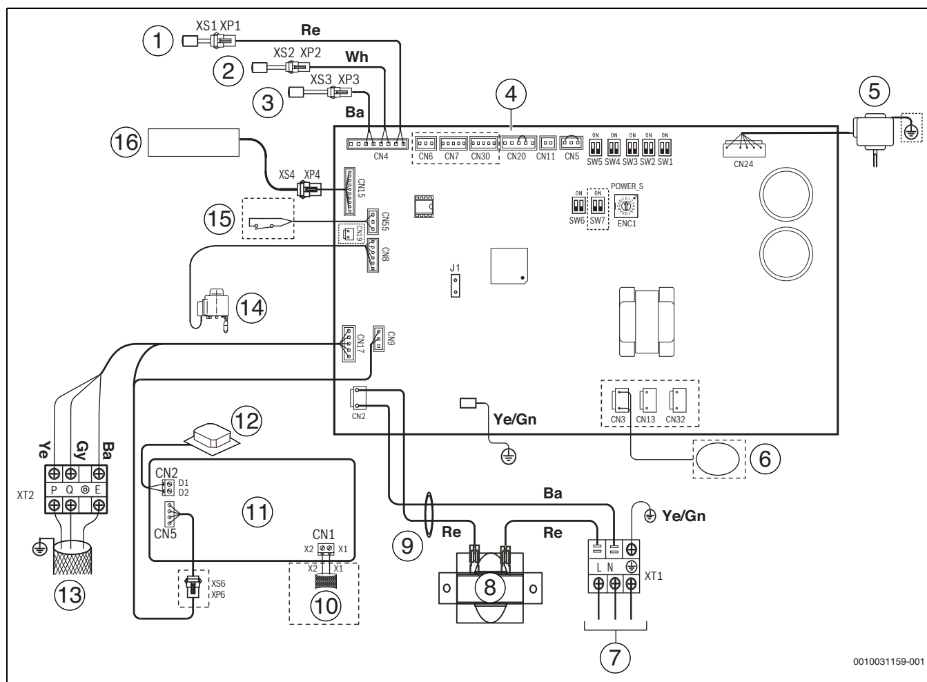
Рис. 47 Электропроводка, прототип 71–80
