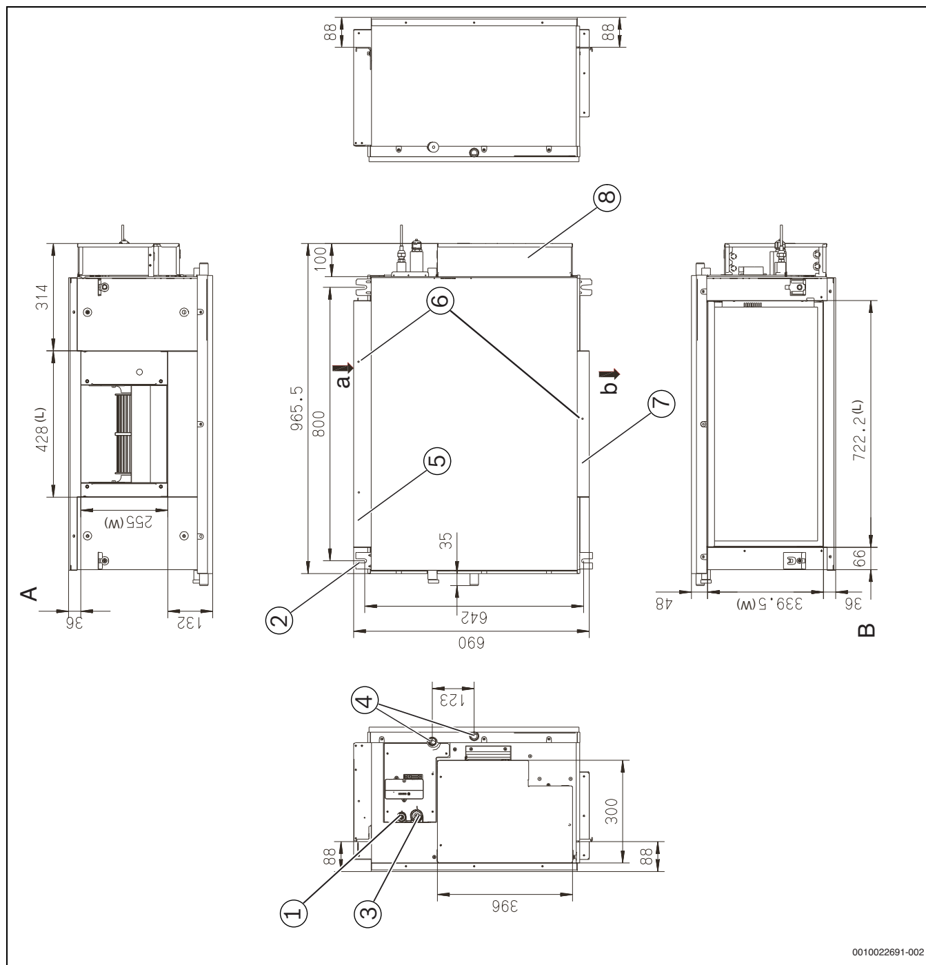
Рис. 9 Размеры прототипов: AF-DH 71-1, AF-DH 80-1, AF-DH 90-1, AF-DH 112-1
