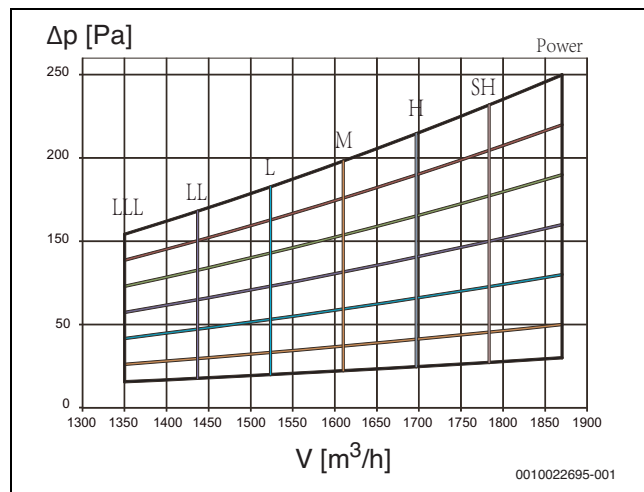
Рис. 25 AF-DH 112-1
