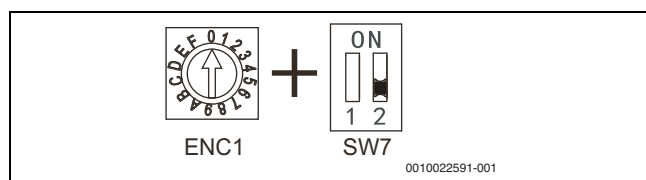
Рис. 42 ENC1 + SW7_2
