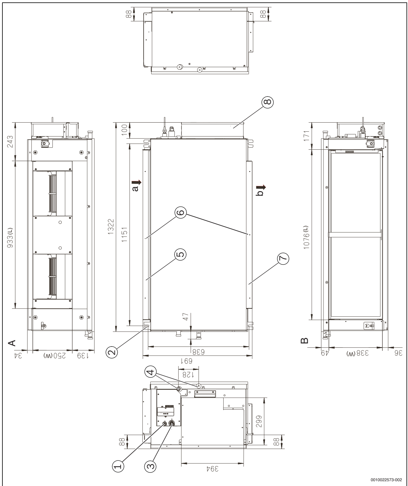
Рис. 10 Размеры прототипов: AF-DH 140-1, AF-DH 160-1
