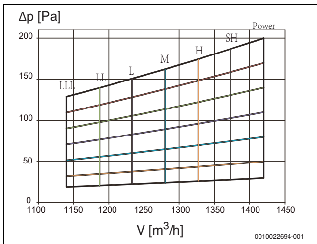
Рис. 24 AF-DH 90-1
