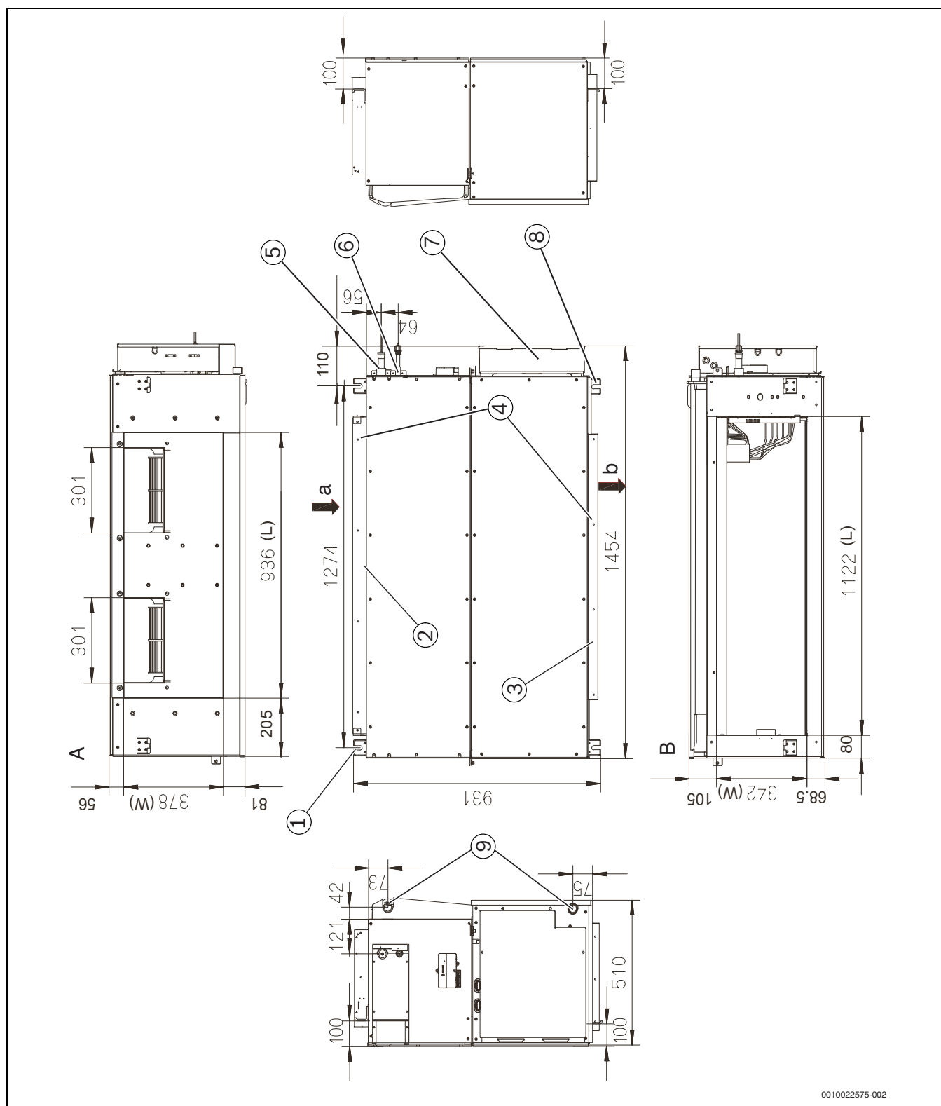
Рис. 11 Размеры прототипов: AF-DH 200-1, AF-DH 250-1, AF-DH 280-1
