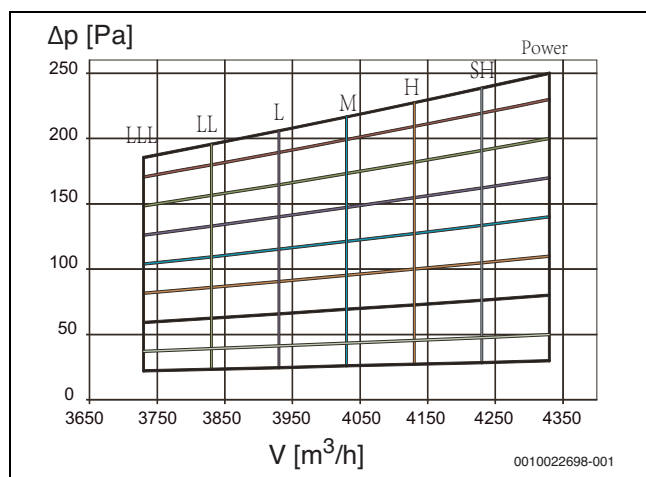
Рис. 28 AF-DH 200-1
