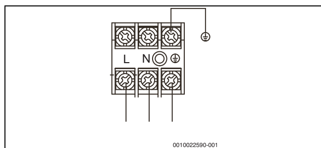
Рис. 35 Входное питание
