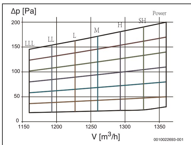
Рис. 23 AF-DH 80-1
