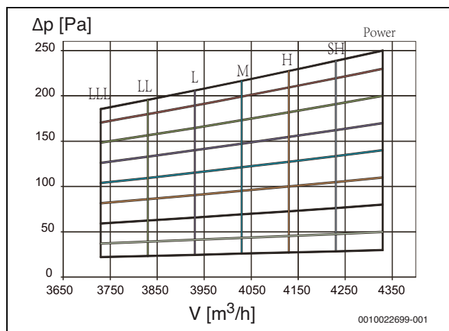
Рис. 29 AF-DH 250-1
