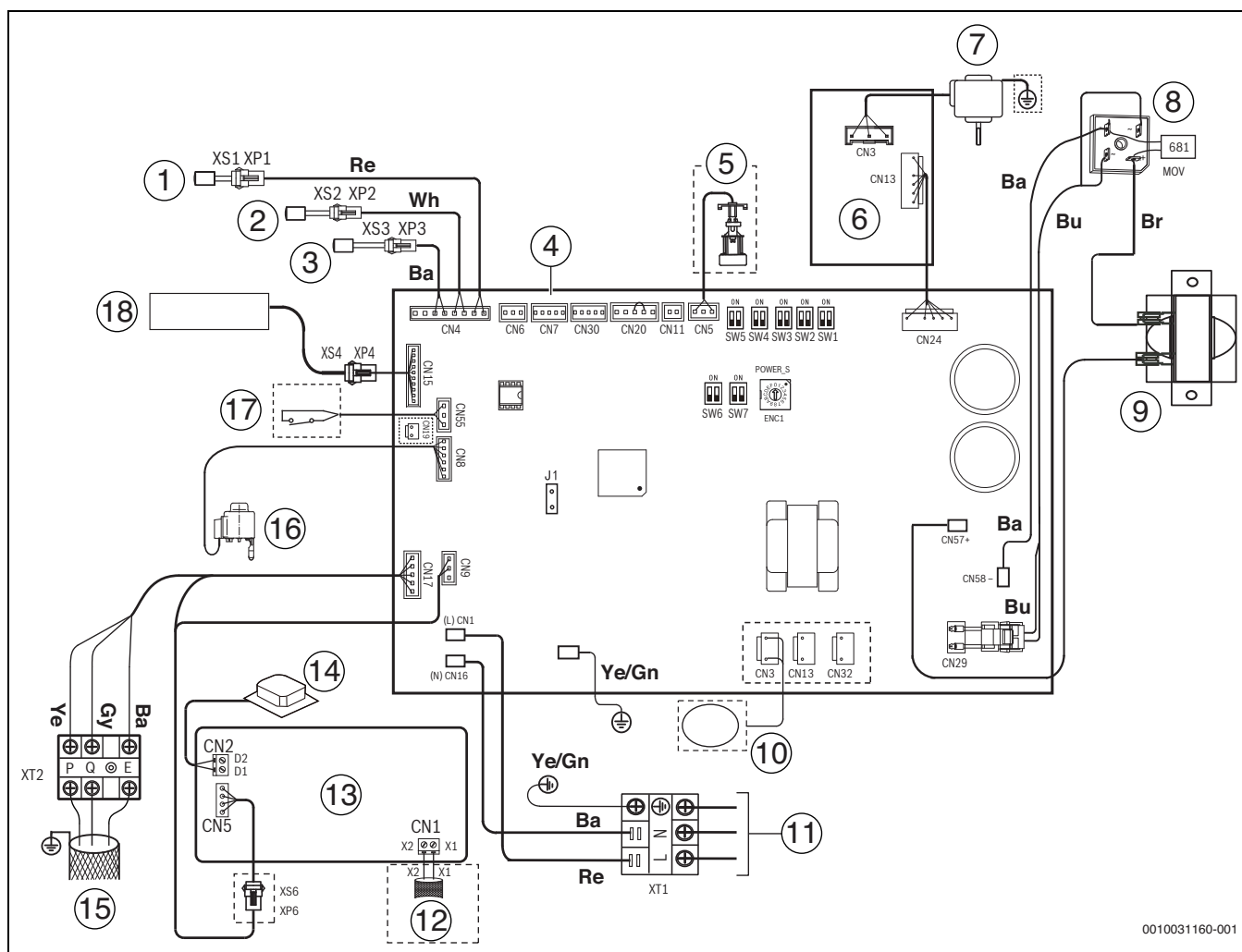
Рис. 48 Электропроводка, прототип 90–160
