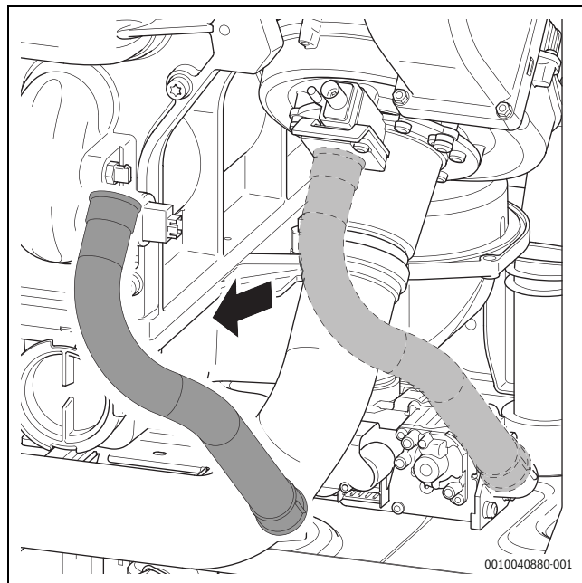
Рис. 35 Отсоединение газового шланга
