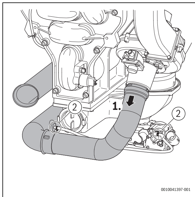
Рис. 36 Демонтаж воздушного коллектора
