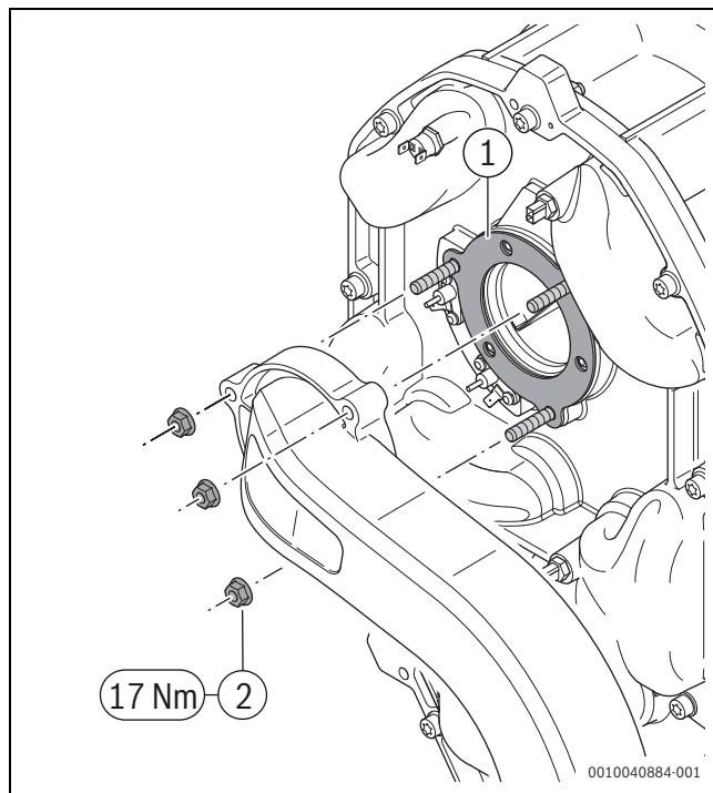
Рис. 43 Установка трубы для смешивания газа и воздуха
