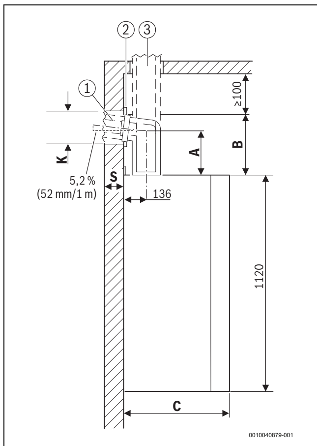
Рис. 4 Вид сбоку [мм]
