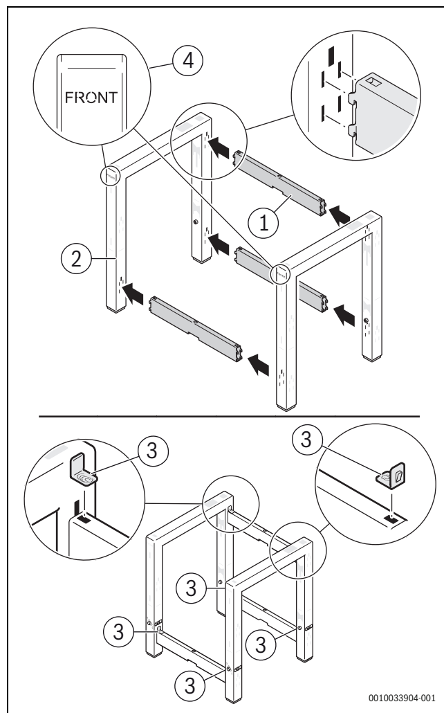
Рис. 8 Установка рамы
