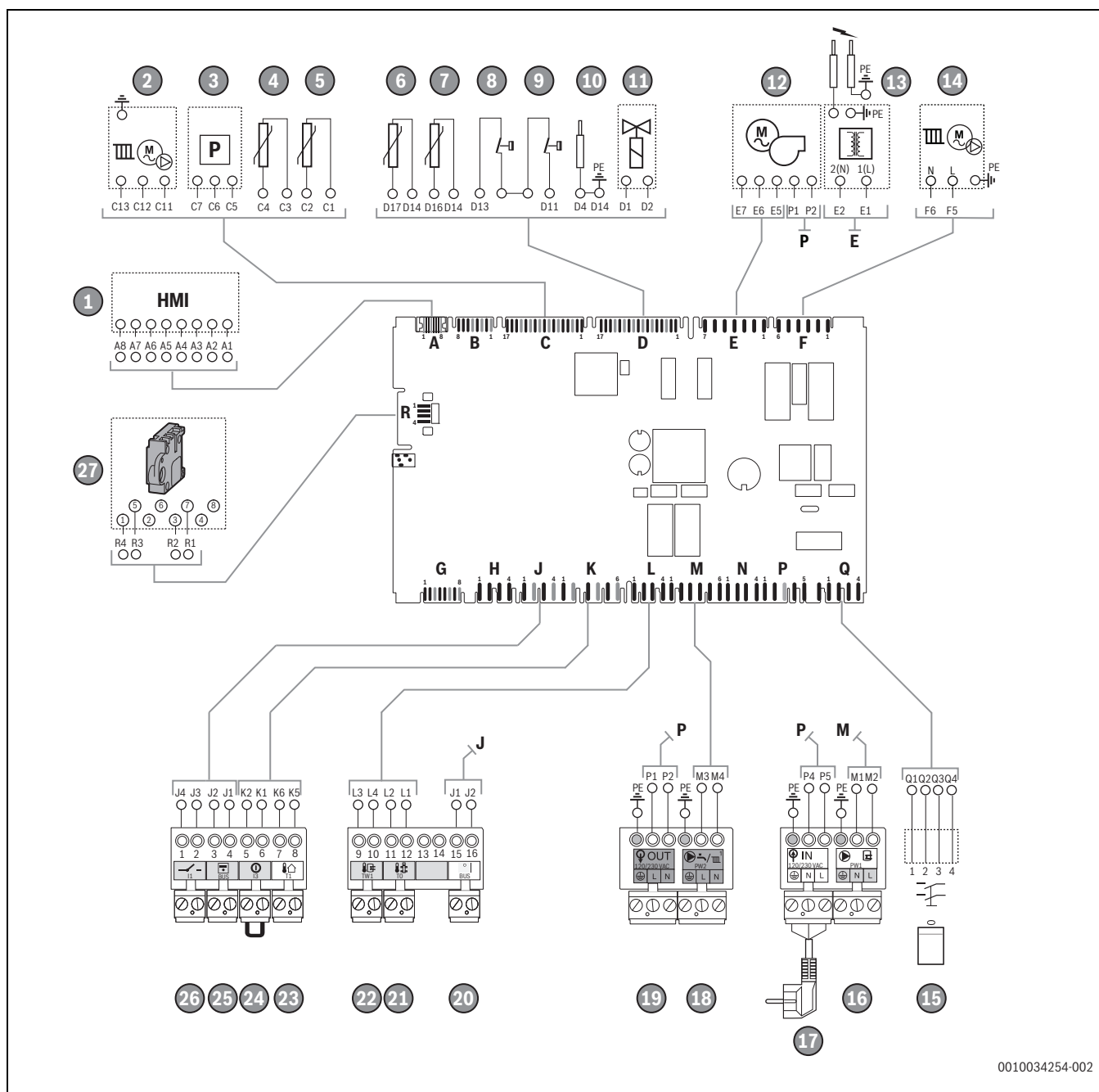
Рис. 49 Электрическая схема
