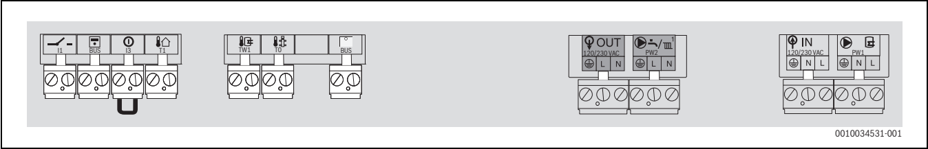
Рис. 23 Обзор штепсельной колодки
