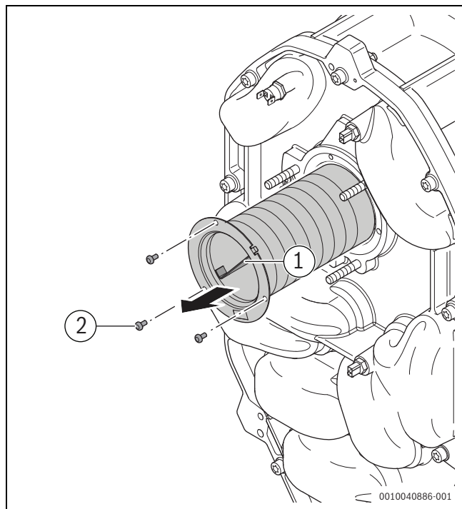
Рис. 38 Разборка горелки
