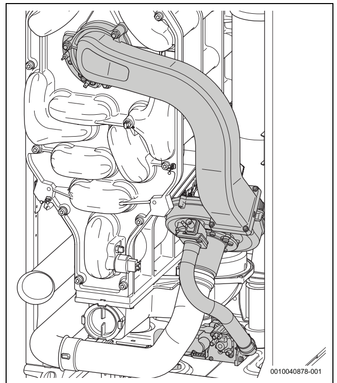
Рис. 33 Контрольные осмотры газовой ramпы
